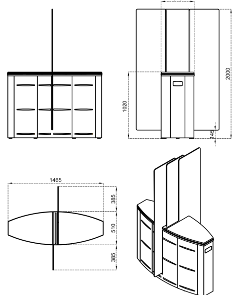
SG 90 T-C Cam Kanat Yüksekliği : 2000 mm
