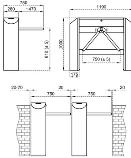
Ölçüler (mm)
