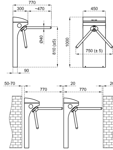
Ölçüler (mm)
