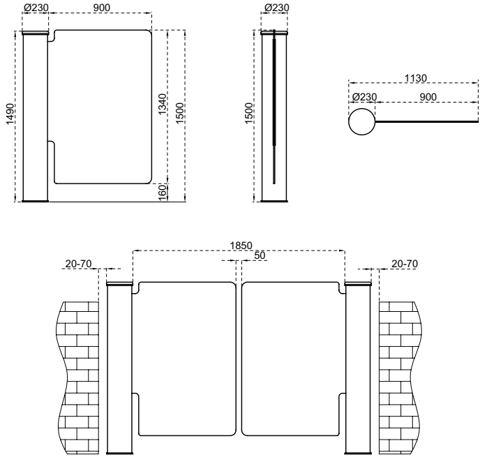
Ölçüler (mm)
